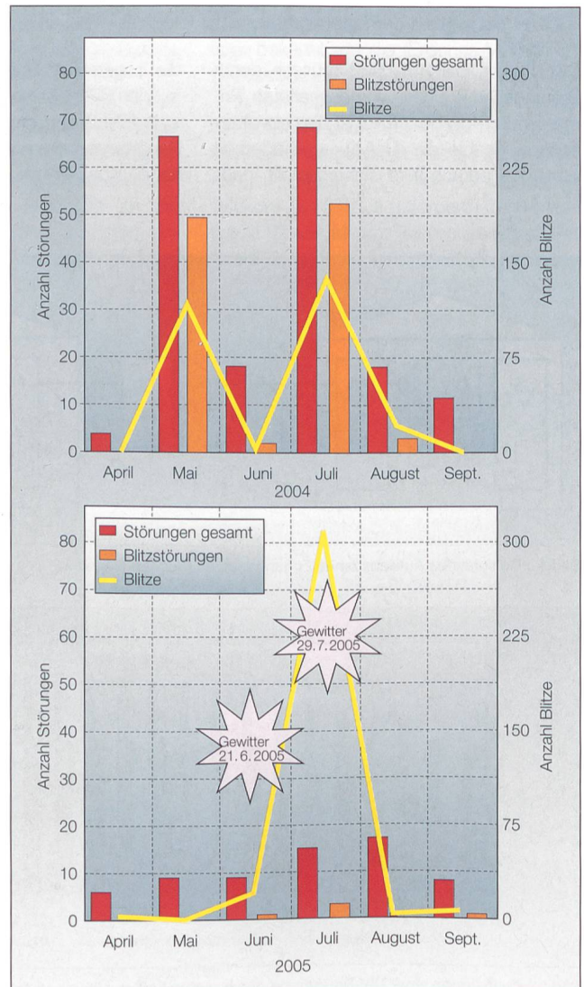
Bild 5 Erfolg der Störungsreduzierung durch Beseitigung von Mängeln im TK-Netz und Potenzialausgleich.
