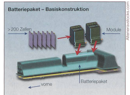
Bild 6 Aufbau und Konstruktion des Chevrolet-Volt-Batteriepakets. Deutlich erkennbar ist die massiv ausgeführte Gestaltung des Batteriepakets zum Fahrgastraum (Panzerung).
