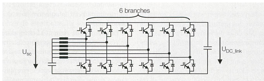
Figure 8 Convertisseur DC/DC bidirectionnel multibranches.
