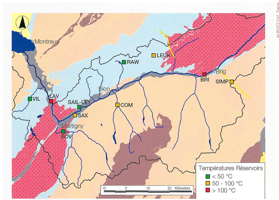
Figure 4 Dans la vallée du Rhône, le sud-ouest et le nord-est disposent des zones les plus favorables pour l'implantation de puits géothermiques et la valorisation de la chaleur.
