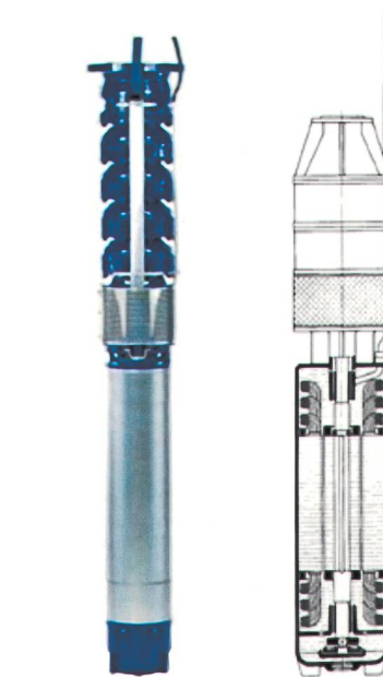
Bild 1 Unterwasser-Motorpumpe [1].
