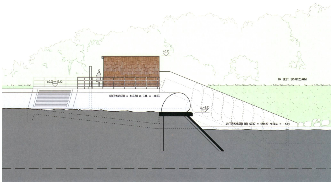
Querschnitt des Kleinwasserkraftwerks mit Wasserkraftschnecke und Fischeaufstiegshilfe.
