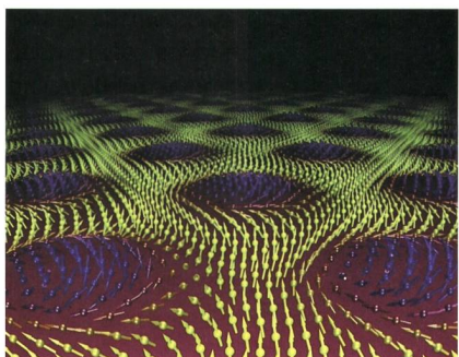
Ein Gitter aus magnetischen Wirbelstrukturen, sogenannten Skyrmeionen.
