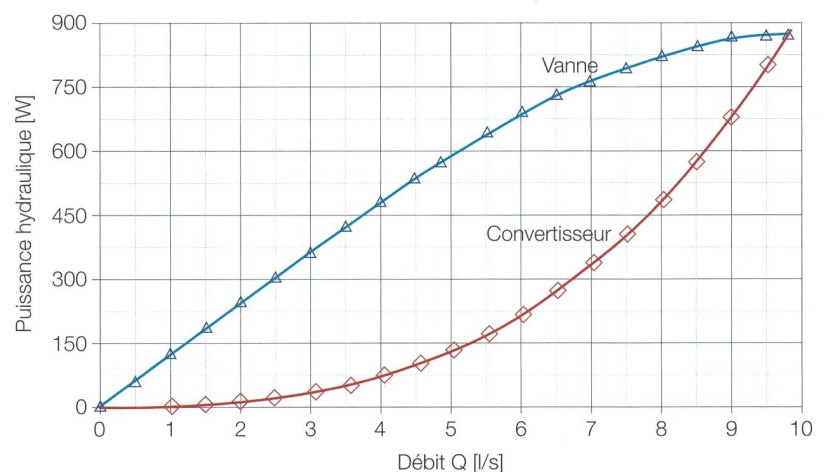
Figure 4 Puissances hydrauliques fournies.
