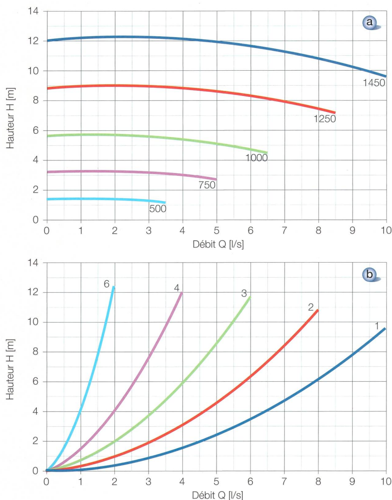
Figure 2 Caractéristiques H(Q) mesurées.
