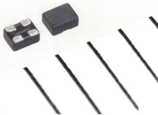
Die Abmessungen in der EIA-Gehäusegrösse 0806 sind 0,85 x 0,65 x 0,40 mm.
