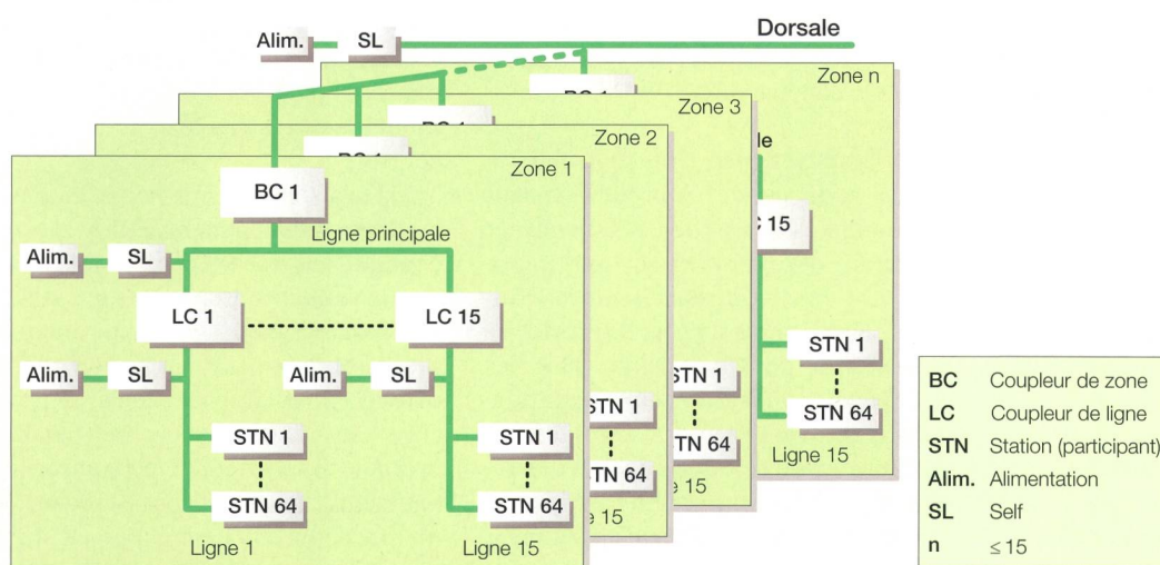
Figure 1 Le réseau EIB/KNX est décomposé en zones, lignes et composants. La paire torsadée nécessite des blocs d'alimentation à différents endroits pour fournir l'énergie nécessaire aux composants.
