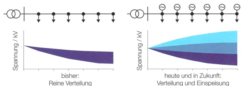
Bild 3 Veränderung der Aufgabe der Spannungshaltung in Verteilungsnetzen bei Zunahme dezentraler Erzeugung (schematisch).
