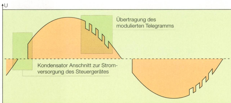
Bild 7 Störungsarme Dimmerfunktion durch Signalübertragung auf der Netzleitung vom Steuergerät zur LED-Vorschaltelctronik nach Ledotron-Standard.
