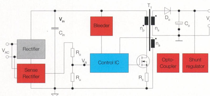
Bild 1 Prinzip eines LED-Vorschaltgerätes.
