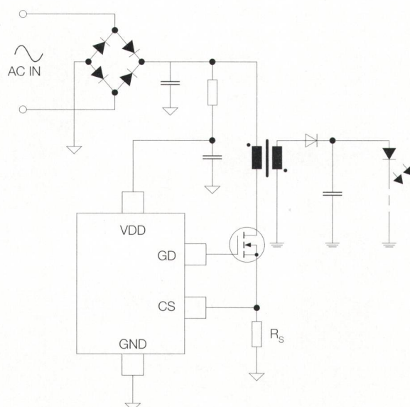
Bild 3 Einfachstes LED-Netzvorschalteschaltungsapplikation mit hohem Leistungsfaktor ohne Dimmbarkeit (Firma LIS, Shanghai, China).
