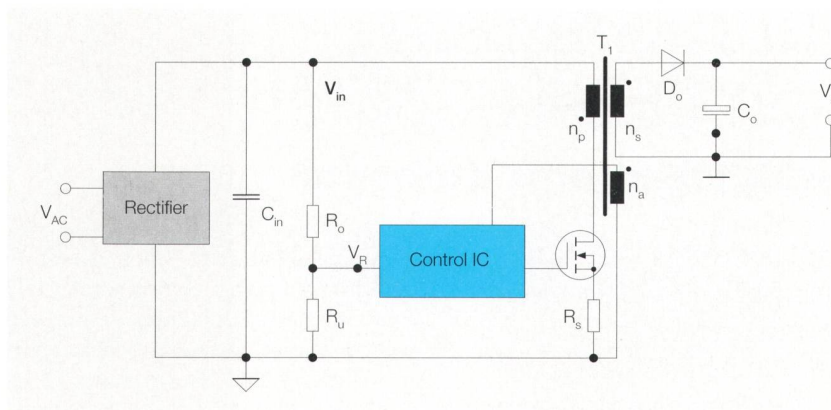
Bild 2 Einfaches Blockschaltbild eines LED-Netzvorschaltes ohne zusätzliche Funktionsblöcke unter Einhaltung eines hohen Leistungsfaktors ( PF > 0,95 ) und Dimmbarkeit mit Phasendimmern (Bleeder nicht gezeigt).
