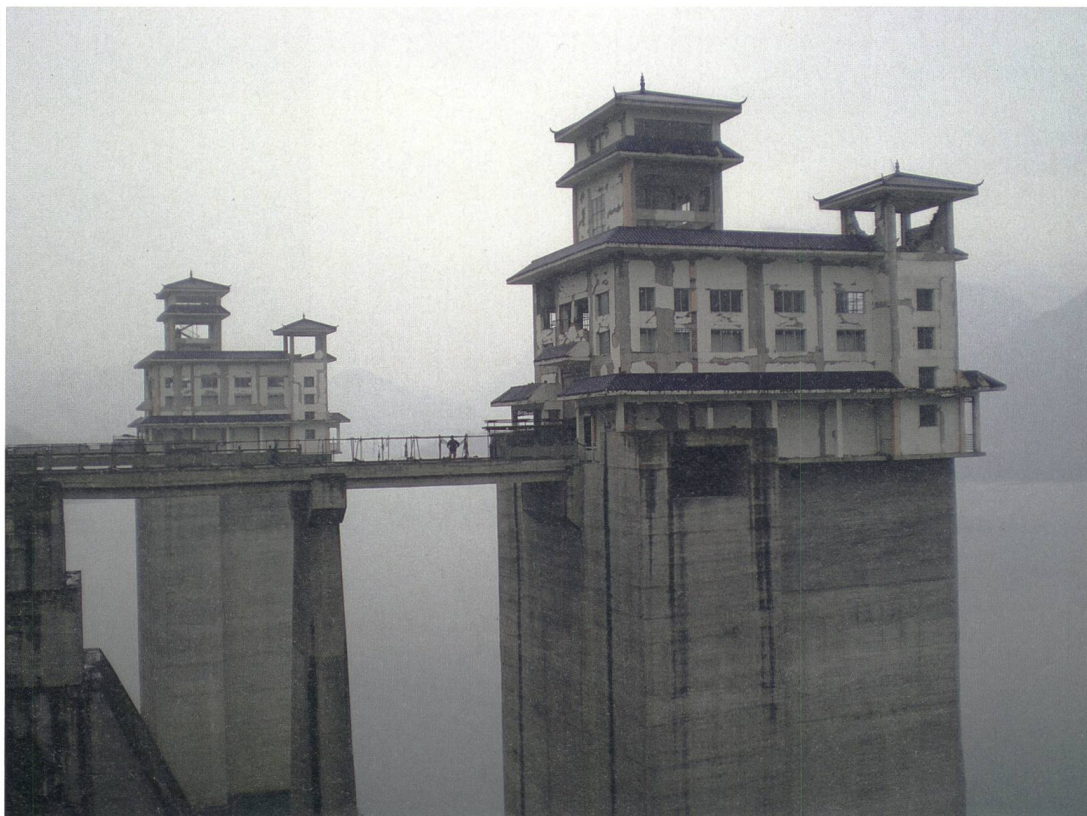
Bild 2 Einlaufbauwerke für die Zipingpu-Stauanlage mit beschädigten Bedienungsgebäuden (Wenchuan-Erdbeben 2008, Sichuan, China).
