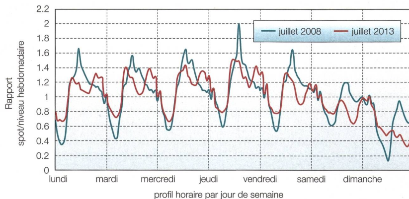
Figure 3 Évolution du profil hebdomadaire du spot allemand en été.
