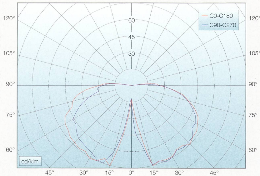
Bild 4 Lichtstärkeverteilungskörper (LVK) einer Gasauflaufleuchte in 2 Achsen radial gemessen.
