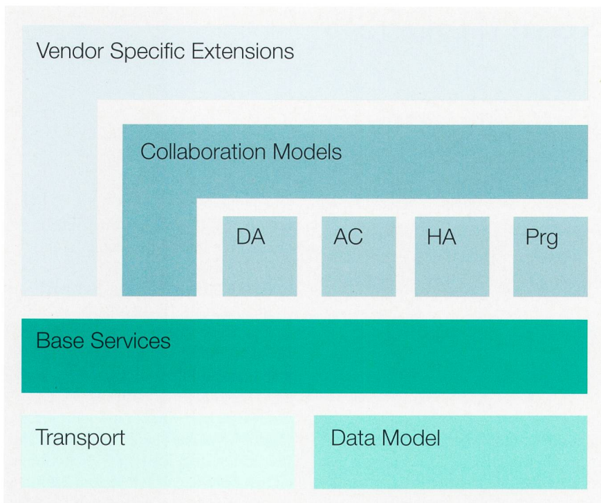
Bild 2 Das PLCopen-Profil von OPC-UA ist ein Vertreter eines auf den Basismechanismen DA, AC, HA, PRG basierten Collaboration-Modells.
