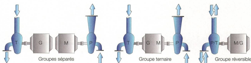
Figure 5 Différentes architectures de groupes de pompage-turbine.
