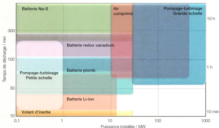
Figure 2 Différentes solutions de stockage en fonction de la puissance requise et du temps de décharge.
