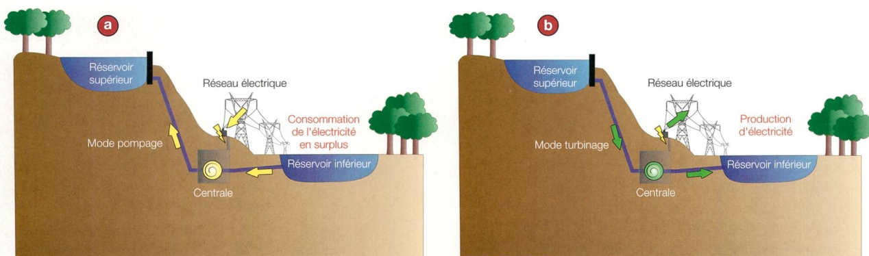
Figure 3 Principe du pompage-turbinage : en mode pompage (a) et en mode turbinage (b).
