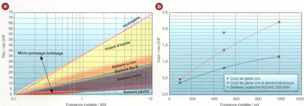
Figure 7 Comparaison des coûts d'investissement des différentes solutions de stockage à petite échelle d'une puissance inférieure à 10 MW (a) et coûts de la centrale de pompage-turbinage d'Arbaz pour 100 kW, 500 kW et 1 MW en comparaison avec une autre solution de stockage de 500 kW (b).
