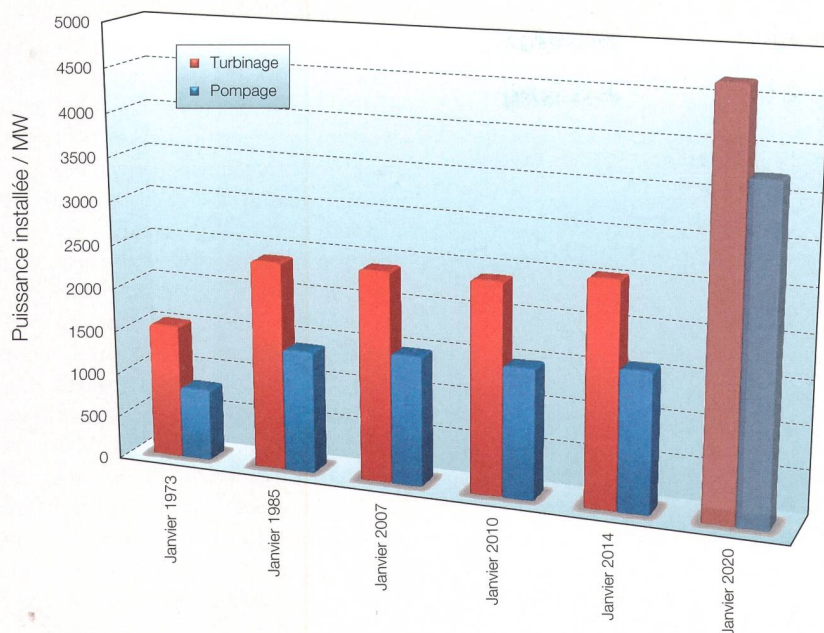
Figure 4 Statistique de l'évolution de la puissance installée en turbine et en pompage en Suisse depuis 1973 jusqu'en 2020 (ont été considérés dans la statistique les ouvrages utilisant les mêmes réservoirs et/ou les mêmes conduites pour les deux modes de fonctionnement) [5].
