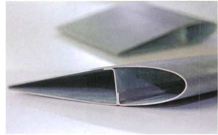
Rotorblatt aus 1,0 mm Stahlblech mit integrierter, gekanteter Verstärkung.
