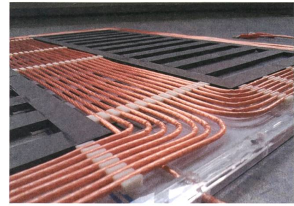
Spulensystem zum induktiven Laden von E-Fahrzeugen.
