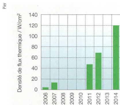
Figure 2 Évolution de la densité de flux thermique.
