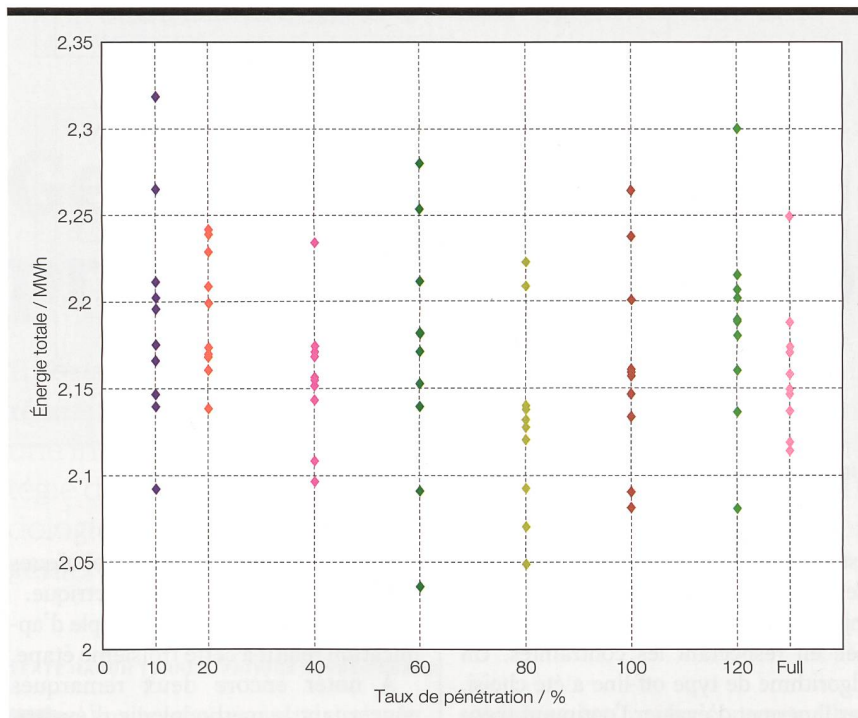
Figure 3 Énergie totale consommée par le réseau électrique.
