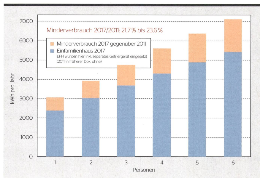
Bild 2 Typischer Haushalt-Stromverbrauch, Einfamilienhäuser, Vergleich mit 2011.
