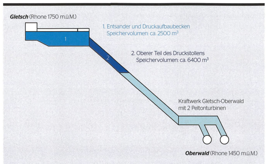
Bereiche, die als Speicher genutzt werden können (nicht massstabsgetreu): Entsanderbecken, Druckaufbaubecken sowie oberer Teil des Druckstollens.
