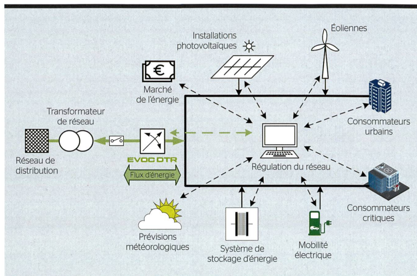
Figure 4 Vue d'ensemble de réseaux intelligents avec le régulateur électronique de tension EVOC-DTR.
