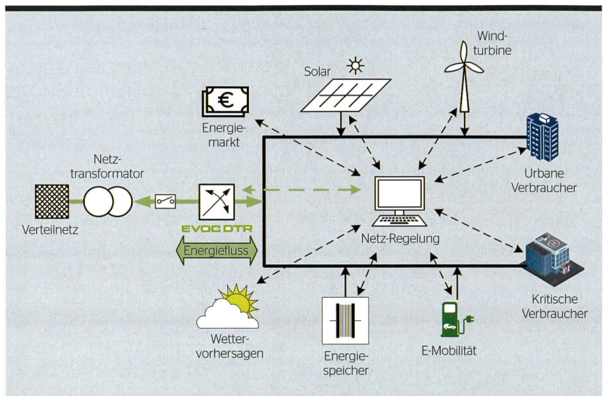
Bild 4 Übersicht von Smart Grids mit dem elektronischen Spannungsregler EVOC-DTR.
