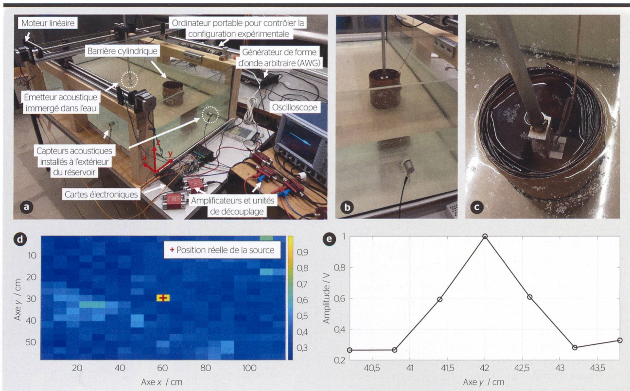
Figure 3 a) Configuration expérimentale, b) vue en perspective, c) vue de dessus de l'émetteur acoustique à l'intérieur de l'obstacle métallique cylindrique multicouche, d) distribution normalisée de la pression maximale sur un plan horizontal du réservoir d'eau à z=13 cm, et e) pression normalisée pour un balayage à l'intérieur de l'obstacle métallique.
