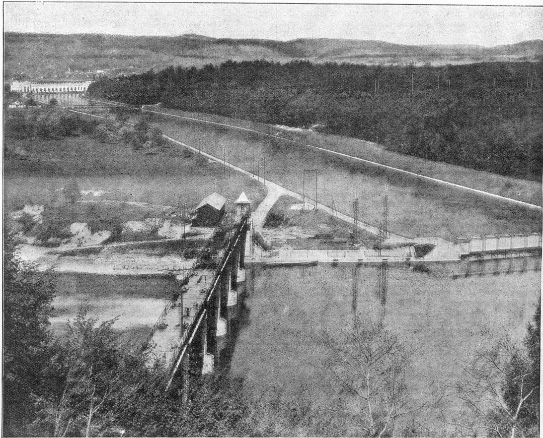
Die Kraftwerke Beznau-Lönsch bei Baden (Kanton Aargau) mit Kanal, Stauwehr, Turbinen-, Kessel- und Schalt haus.
