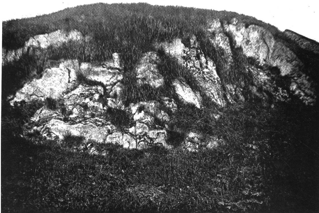
No. 10. Die offene Felsflora geht in die geschlossene Wiesenflora über durch die Tätigkeit von Festuca varia . Felskopf an der Oberalpstraße.
