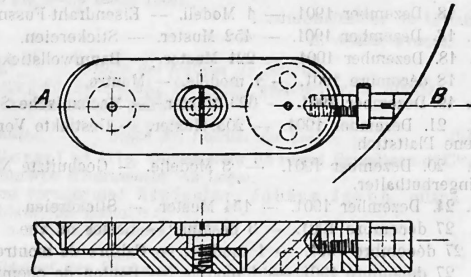
Coupe: A-B.
