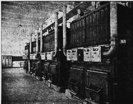
Großheizwerk mit 8 OERTLI-Zwillingsbrennern an vier SULZER-Taschenkesseln
