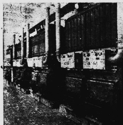
OERTLI-Industrie-Oelfeuerungsanlage mit Zwillingsbrennern an Sulzer-Taschenkesseln (Heizzentrale Flughafen Kloten).
