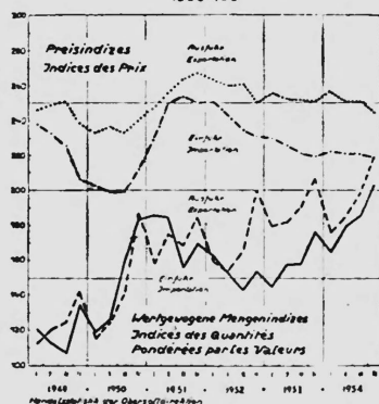
Russenhandelsindizes Indices du commerce extérieur 1938=100
