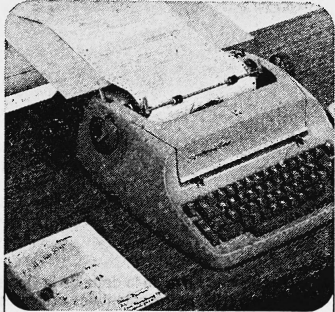
Der maschinenlesbare Schreibstreifen ruft die gewünschten Texte vom Magnetbandspeicher ab. Blitzschnell, mit über 1,2 Millionen Zeichen/min erfolgt die Selektionssteuerung.
