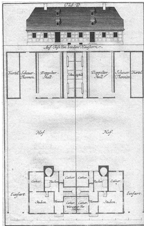
Abb. 22, 23: Johann David Steingruber, Abdruck eines Hoch-Fürstlich-Brandenburg-Onolzbachischen Ausschreibens [...], Augsburg: Hofbuchhändler, 1753, Tafel P, Musterentwurf für ein doppeltes Bauernhaus und ein doppeltes Ökonomiegebäude mit Stall und Scheune und o.S., Kostenvoranschlag für Materialien und Arbeitslohn einer neuen Scheune mit Wagenschopf
