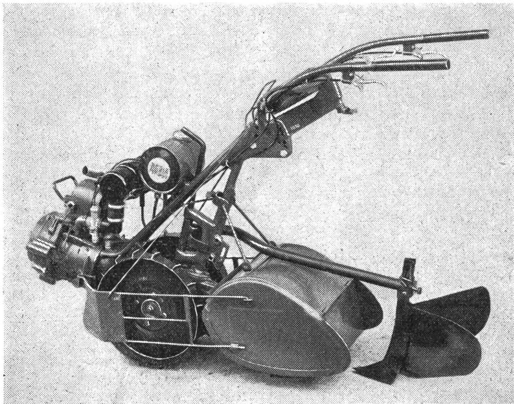
AGRIA — Universal 5 PS 200 ccm als Bodenfräse mit Häufler und Blattabweiser.
