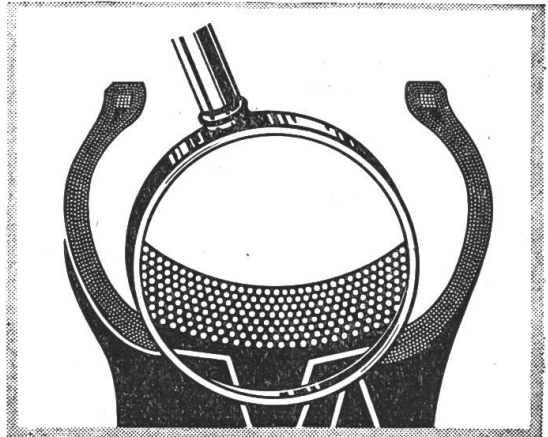
Doppellagen als Schlagschutz. Zwei besondere Gewebelagen, welche die stärksten Schläge zu tragen vermögen, schützen wirkungsvoll den Cord-Unterbau.
