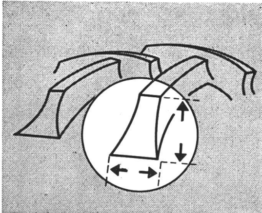
Wuchtigere, kräftigere Schultern verbessern den Laufflächenkontakt mit dem Grund und erhöhen die Griffigkeit. Die Abnützung wird gleichmässig und die Lebensdauer grösser.
