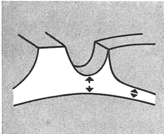
Die solid verstrebt Basis verhindert das übermässige Durchbiegen der Stollen. Das Aufprallen der Stollen-Enden wird dadurch ausgeschaltet.
