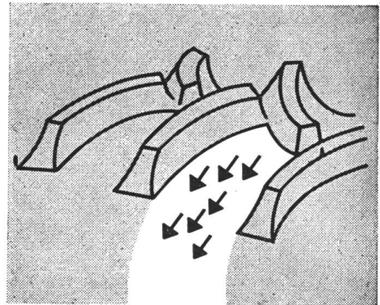
Bewegliche Profil-Kanäle. Zur Verhinderung des Erdstaus und zur Erleichterung des Erdabflusses.
