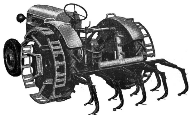
Meili-Giterräder und Kultivator
