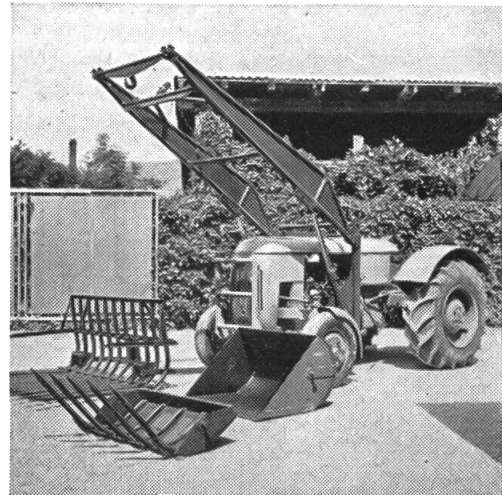
Frontlader Wittenburg-Vevey
