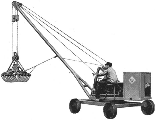
Mistladekran Mengele
