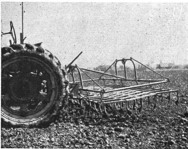
Vogel-Ackeregge an Dreipunktbaurahmen
