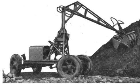
Atlas-Ladegerät der Fa. AIMSA, Genf
