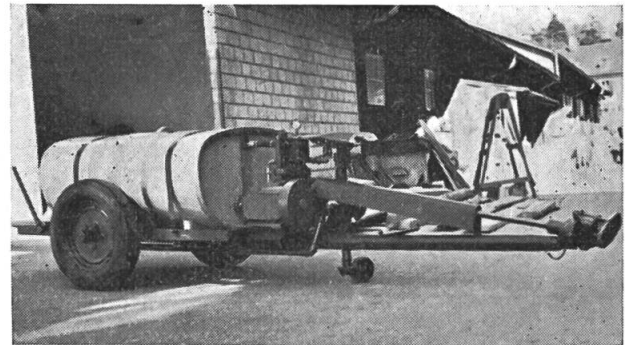
Royal-Hochdruck-Spritze für Zapfwellenantrieb
