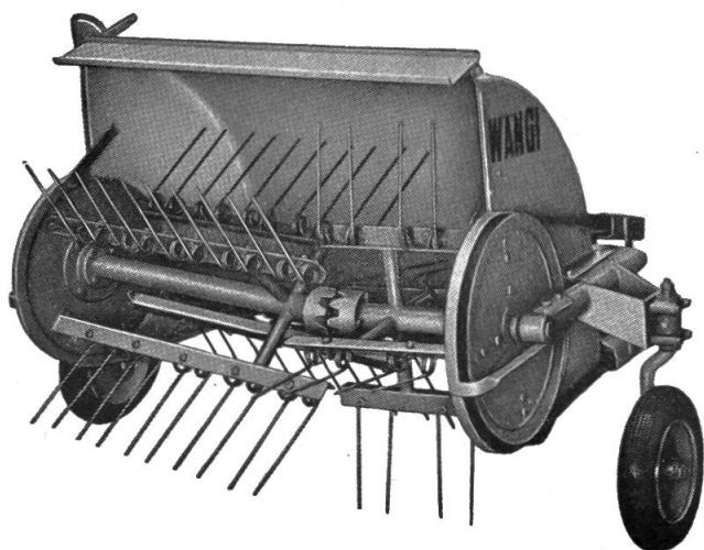
oben: Zapfwellen-Wender «Wängi»
