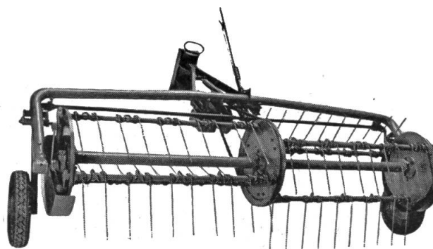
oben: Zapfwellen-Wender «Wängi»
