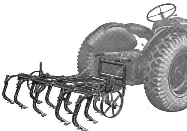
Dreipunkt-Anbaurahmen mit Kultivator «Althaus»
