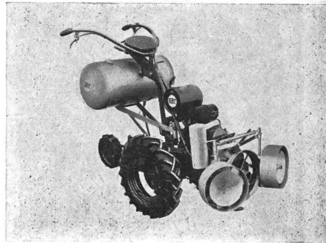
Abb. 8: Doppelturbogerät zum Pflanzenschutz und zur Schädlingsbekämpfung, zum Anbau an Agria, Typ 1600, 5 PS.
