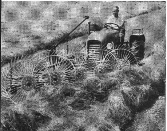
Rotorrechen für Frontmontage oder als gezogene Maschine
