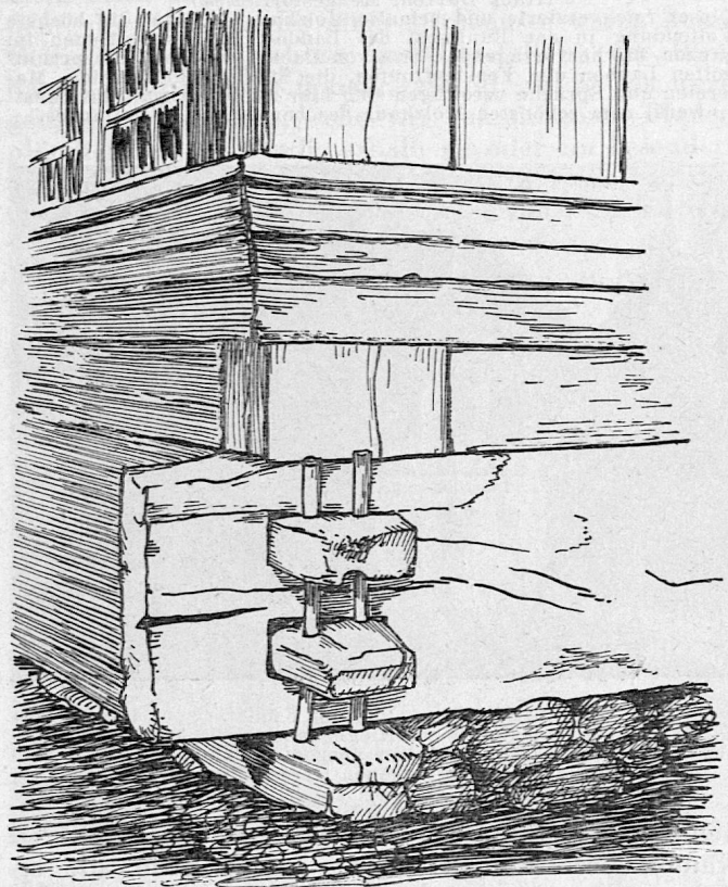
Die Schwelle eines alten Hochstudhauses (Richigen b. Worb). Die dicken Eichenschwellen sind an ihren Enden mit Holznägeln verzäpft. Auf der Schwelle ruht das ganze gewaltige Holzhaus. Zeichnung von P. Howald
