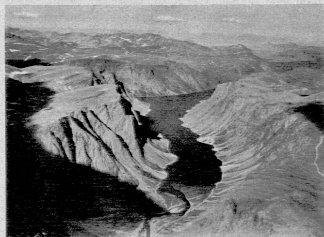
Labrador, Fjord in der Sagleyk Bay. Die Aufnahme zeigt den Gegensatz zwischen leicht gewellter Hochfläche und tief eingeschnittenem und glazial überformtem Taltrög besonders deutlich.
