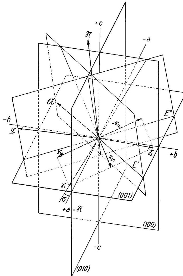
Fig. 13. Zur Berechnung der Auslöschungsschiefe auf P (001) von Albit, bezogen auf die Spur von M(010). Die beiden Vektoren r_1 = [\mathfrak{M}\mathfrak{A}] bzw. r_2 = [\mathfrak{M}\mathfrak{B}] stehen normal auf den durch die Normale \mathfrak{N} auf P(001) und die optischen Achsen \mathfrak{A} bzw. \mathfrak{B} aufgespannten Ebenen E' bzw. E'' . Die gesuchten Schwingungsrichtungen \mathfrak{S}_1 und \mathfrak{S}_2 werden durch vektorielle Addition bzw. Subtraktion der Einheitsvektoren r_{1_0} und r_{2_0} erhalten. Die Bezugsrichtung \mathfrak{R} , welche der kristallographischen a-Achse entspricht, ist Schnittkante von P(001) und M(010), d. h. es ist \mathfrak{R} = [\mathfrak{M}\mathfrak{N}] . Der gesuchte Auslöschungswinkel \sigma ergibt sich aus dem skalaren Produkt (\mathfrak{S}_1\mathfrak{R}) .
