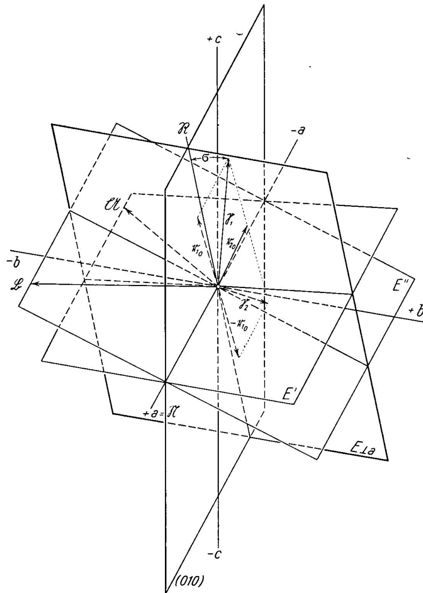
Fig. 14. Zur Berechnung der Auslöschungsschiefe für einen Schnitt \perp a , bezogen auf die Spur von M(010) für Albit. Die beiden Vektoren r_1 = [R\mathcal{A}] bzw. r_2 = [R\mathcal{B}] stehen normal auf den durch die Normale zur betrachteten Fläche \mathcal{R} = a und die beiden optischen Achsen \mathcal{A} bzw. \mathcal{B} bestimmten Ebenen E' und E'' . Die beiden Schwingungsrichtungen \mathcal{S}_1 und \mathcal{S}_2 werden durch vektorielle Addition bzw. Subtraktion der Einheitsvektoren r_{10} und r_{20} erhalten. Die Bezugsrichtung \mathcal{R} ist die Schnittkante der Ebene \perp a mit M(010) , d. h. es ist \mathcal{R} = [R\mathcal{M}] . Der gesuchte Auslöschungswinkel \sigma ergibt sich aus dem skalaren Produkt (\mathcal{S}_1\mathcal{R}) .
