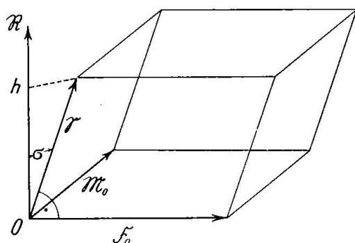
Fig. 11. Der Auslöschungswinkel \sigma ist gleich der Schiefe des durch die drei Vektoren \mathfrak{F}_0 (Einheitsnormalvektor der betrachteten Fläche F ), \mathfrak{M}_0 (Einheitsnormalvektor der Bezugsfläche M ) und \mathfrak{S} (Schwingungsrichtung) aufgespannten Parallelepipeds mit der Grundfläche [\mathfrak{F}_0 \mathfrak{M}_0] .
