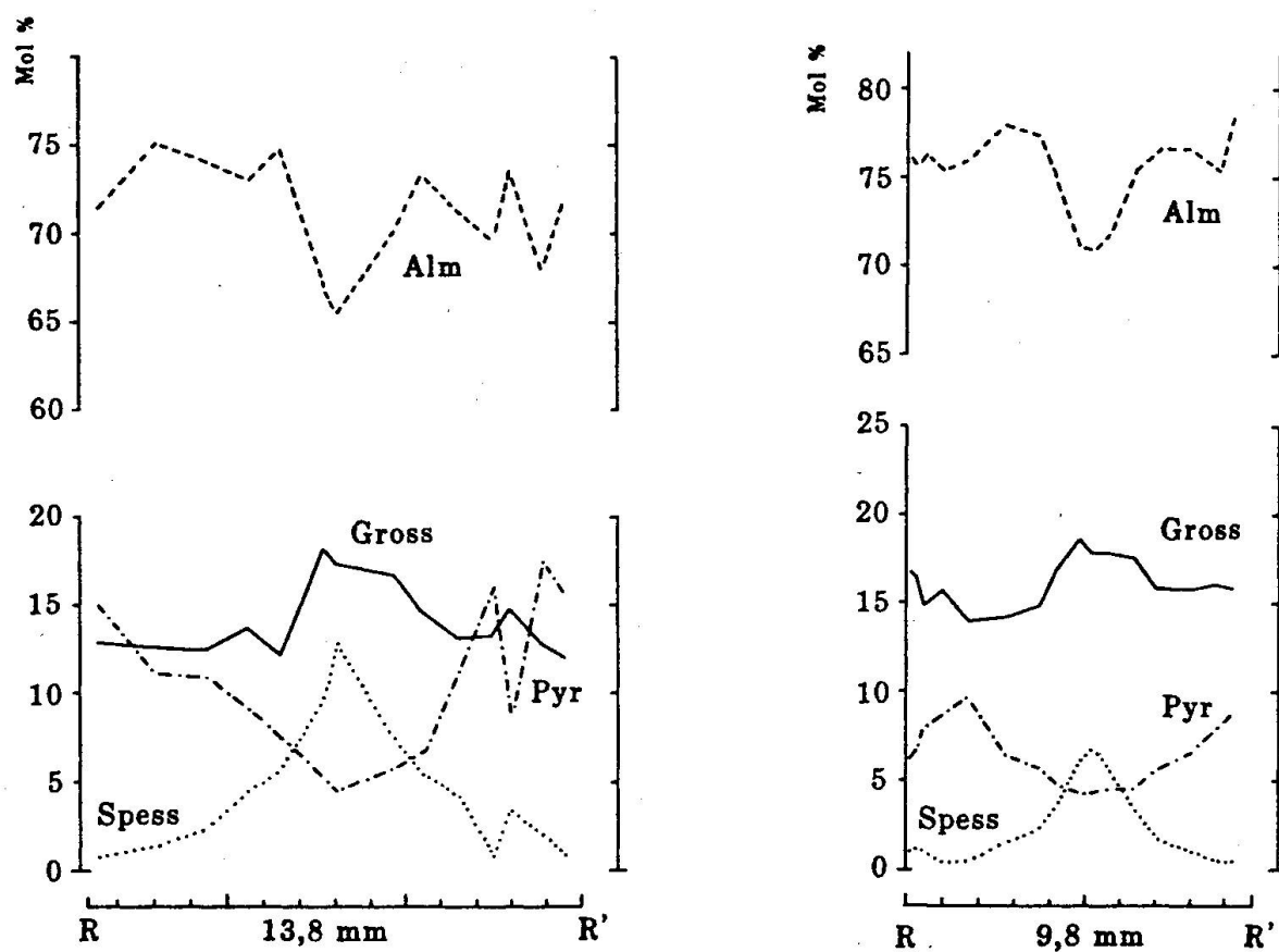
Fig. 1a, b Profils de composition de grenats (microsonde) par le centre, montrant des zonation typiques. Z = centre, R, R' = bords.
