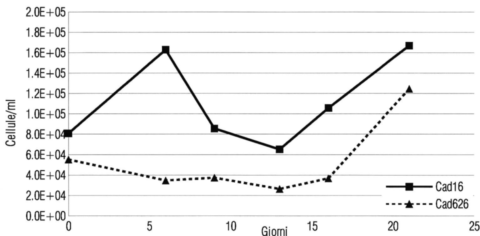
Fig. 6 - Curve di crescita delle cellule nei sacchi per la dialisi posti a 11.5 m. La linea continua rappresenta la crescita di T. syntrophicum Cad16, la linea tratteggiata rappresenta la crescita di D. thiozymogenes Cad626. Al giorno 21 non rileva alcun crollo della cultura anzi le cellule continuano a crescere.
