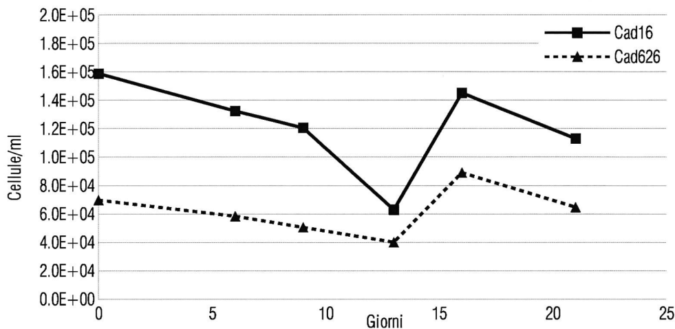
Fig. 7 - Curve di crescita delle cellule nei sacchi per la dialisi posti a 12.5 m. La linea continua rappresenta la crescita di candidato T. syntrophicum Cad16, la linea tratteggiata rappresenta la crescita di D. thiozymogenes Cad626.
