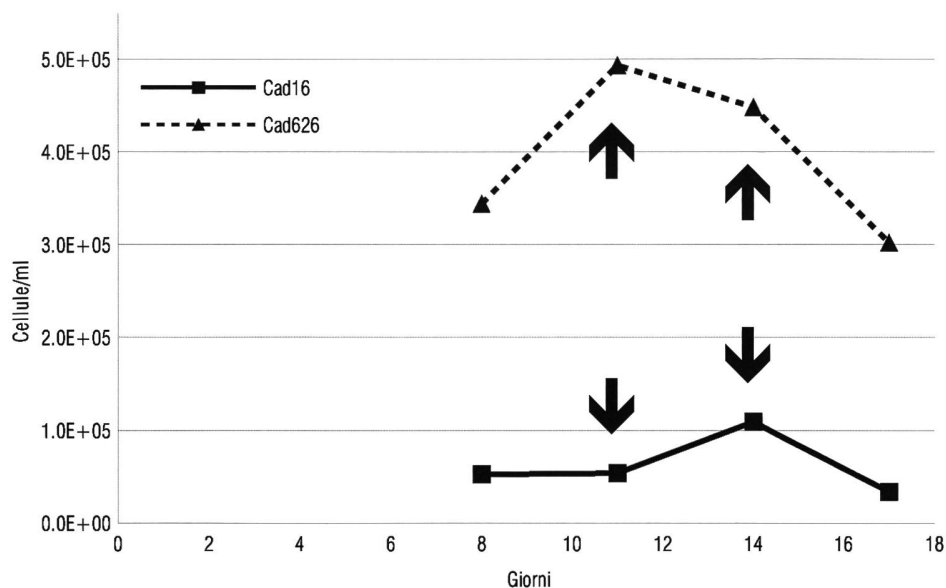
Fig. 11 - Cellule/ml presenti nel terreno misto allestito per la crescita di Cad16 e Cad626 in condizioni di microaerofilia e in presenza di una concentrazione iniziale di solfato pari a 2.0 mM. La linea tratteggiata rappresenta la crescita di D. thiozymogenes Cad626, la linea continua rappresenta la crescita candidato T. syntrophicum Cad16. Le frecce indicano le fasi in cui abbiamo individuato gli aggregati.
