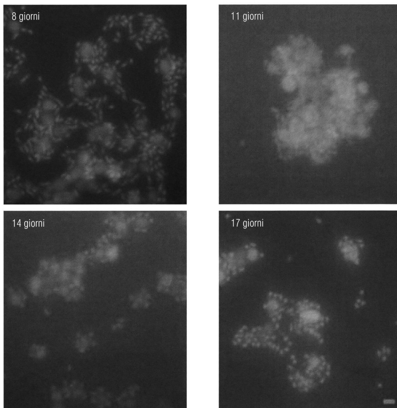
Fig. 10 - Le immagini di microscopia a campo largo mostrano lo sviluppo della crescita delle cellule in condizioni aerobiche e in presenza di una concentrazione iniziale di solfato pari a 2.0 mM. D. thiozymogenes Cad626 presenta una morfologia a bastoncino candidato T. syntrophicum Cad16 presenta una morfologia sferica. La scala è di 2 µm.
