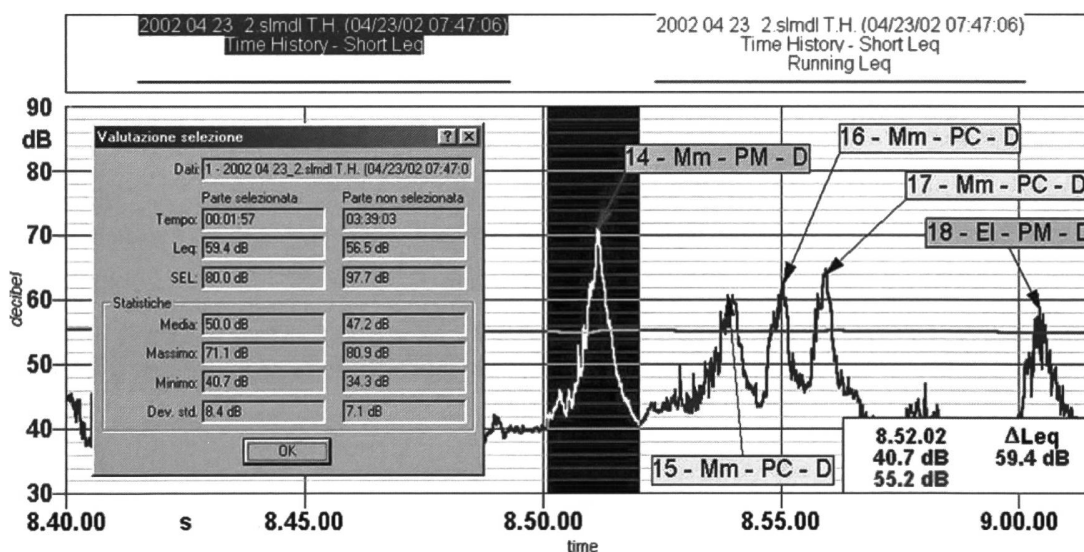
Fig. 2: Esempio di elaborazione effettuata con il software di gestione "Noise & Vibration Works 1.26". L'andamento del SLeq (linea sinuosa) presenta picchi identificabili come il transito di un velivolo utilizzando i dati delle osservazioni su campo. Per ognuno dei picchi presenti nell'immagine sono indicati il numero progressivo giornaliero del volo, il tipo di velivolo (Mm: monomotore; El: elicottero), la pista interessata (PM: pista militare asfaltata; PC: pista civile inerbata), il tipo di movimento (D: decollo). La casella "valutazione selezione" contiene i parametri calcolati dal programma per l'evento selezionato, tra cui MAX e SEL.
