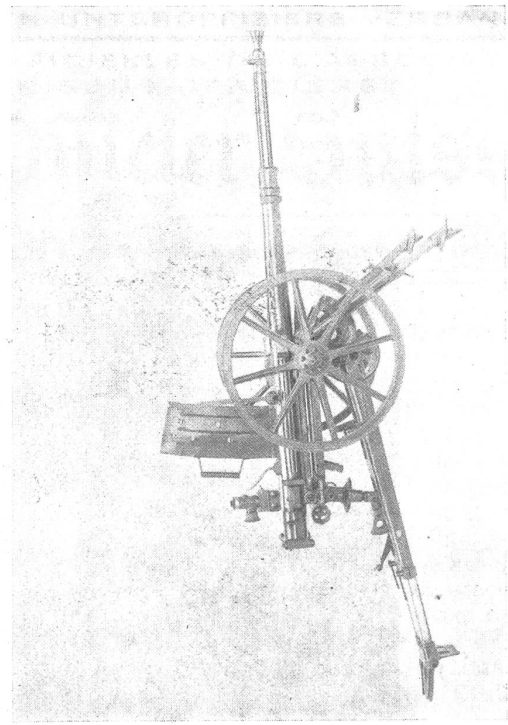
2 cm-Kanone « Oerlikon » in Schiessstellung auf Spreizfüssen mit hochgeschraubten Rädern. Canon de 2 cm « Oerlikon » en position de tir sur appui, roues levées.
