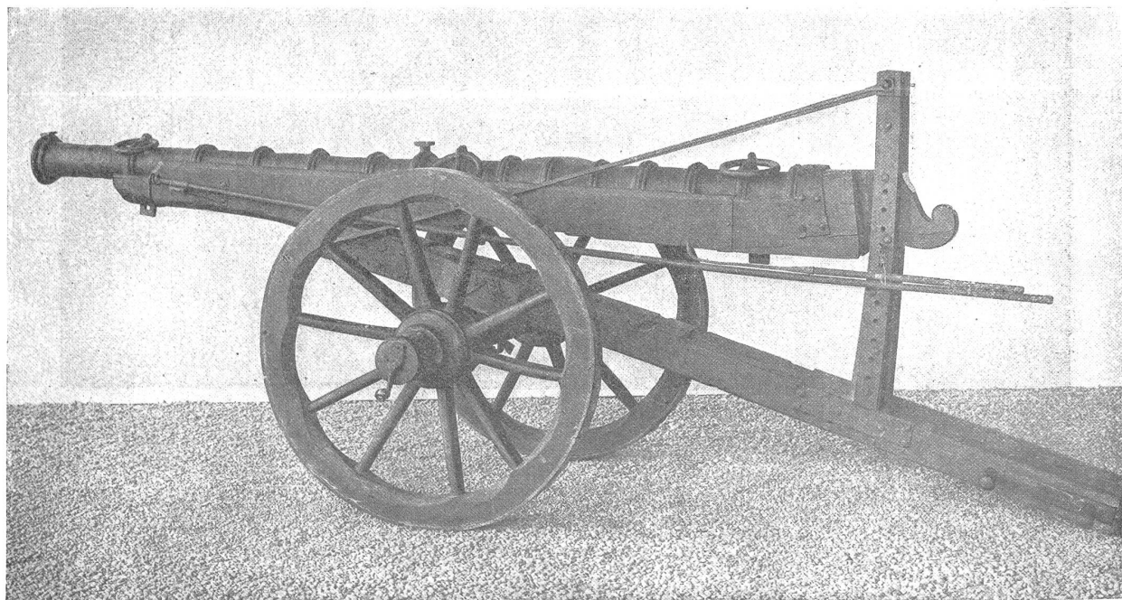
Feldschlange, « Lotbüchse ». Schmiedeisernes Ringgeschützrohr in « Burgunderlafette ». Historisches Museum Neuenstadt. Mitte des 15. Jahrhunderts.
