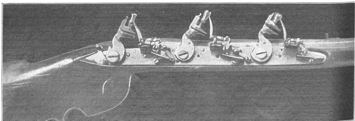
Ein Dreischussgewehr mit Steinschlössern aus der Mitte des 17. Jahrhunderts. — Un fusil à 3 coups (milieu du 17 e siècle).
