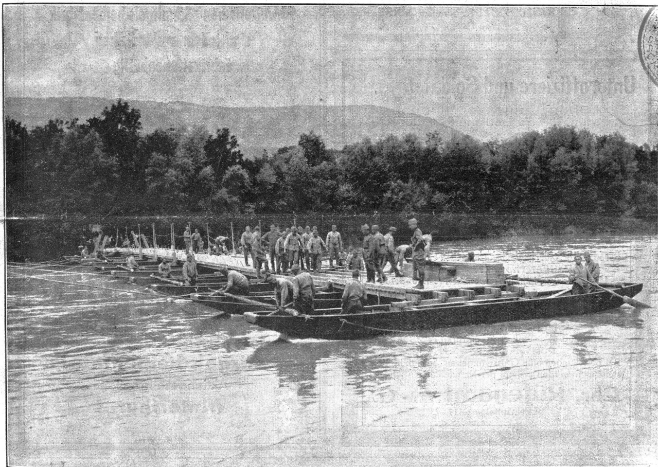
Zusammensetzen einer flussabwärts verlegten Brücke. Einbau eines Brückengliedes. (W.-K. 1928. Pont.-Bat. 2.)
