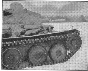
Die Kletterfähigkeit über senkrechte Absätze entspricht in der Regel der Höhe der vordersten Radachse über Boden. Für leichte und mittlere Panzerwagen beträgt sie rund 1 m; ganz schwere Wagen kommen auf 1,7 m. (VIB 1361.)
